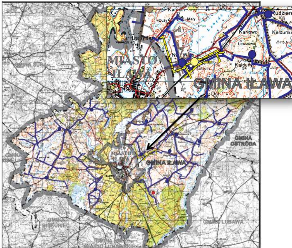
Rysunek 12. Schemat przebiegu istniejącego gazociągu wysokiego ciśnienia relacji Brodnica – Nowe Miasto Lubawskie – Ława przez Gminę Ława
