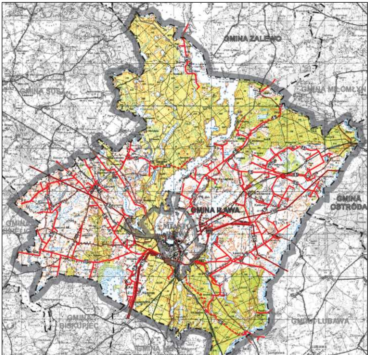
Rysunek 15. Schemat systemu elektroenergetycznego na terenie Gminy Ława
