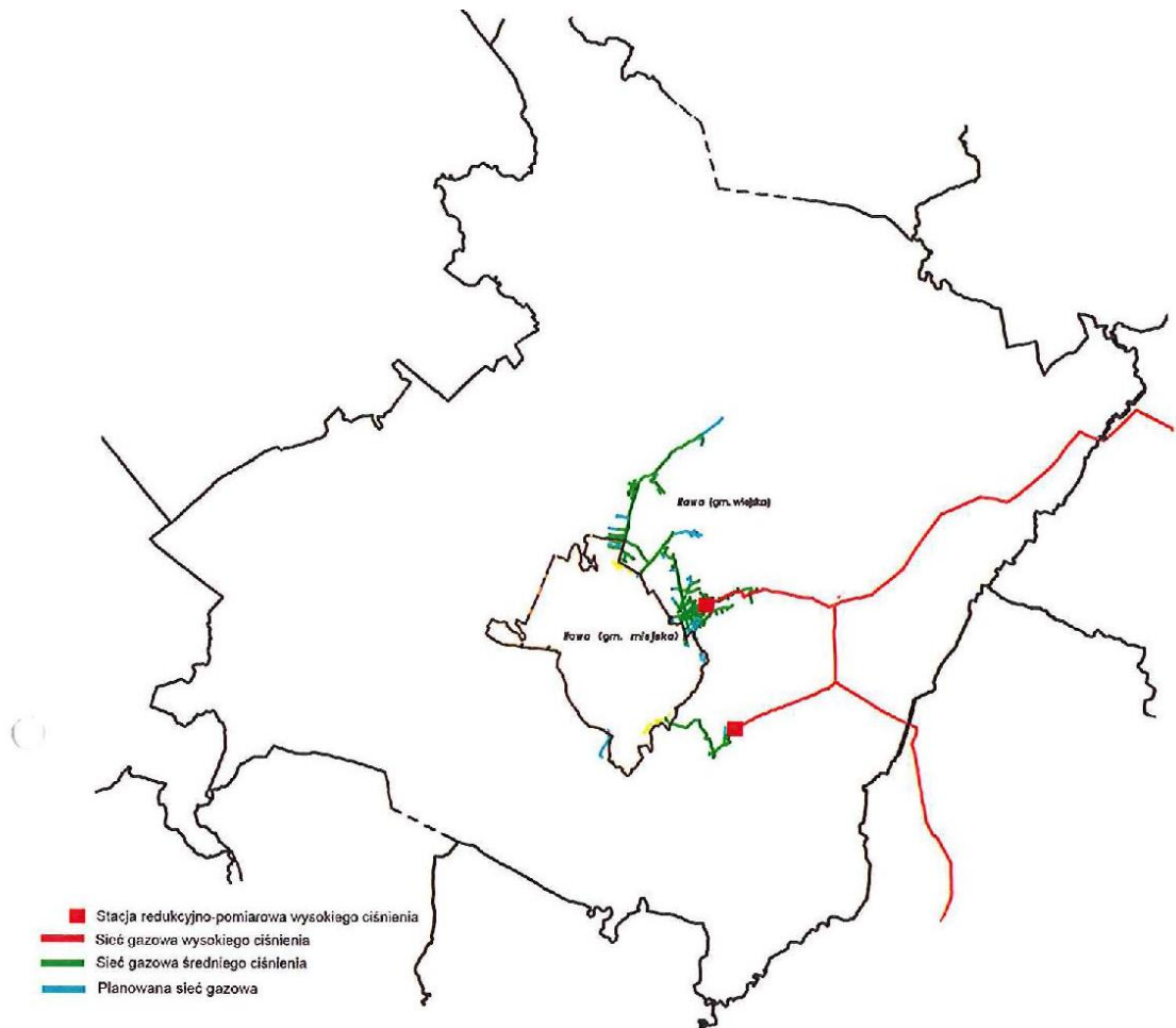
Rysunek nr 14. Schemat sieci gazowej na terenie Gminy Iława
