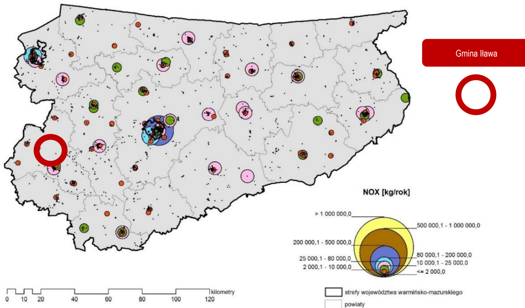
Rysunek nr 16. Lokalizacja punktowych źródeł emisji NOX na obszarze województwa warmińsko-mazurskiego
