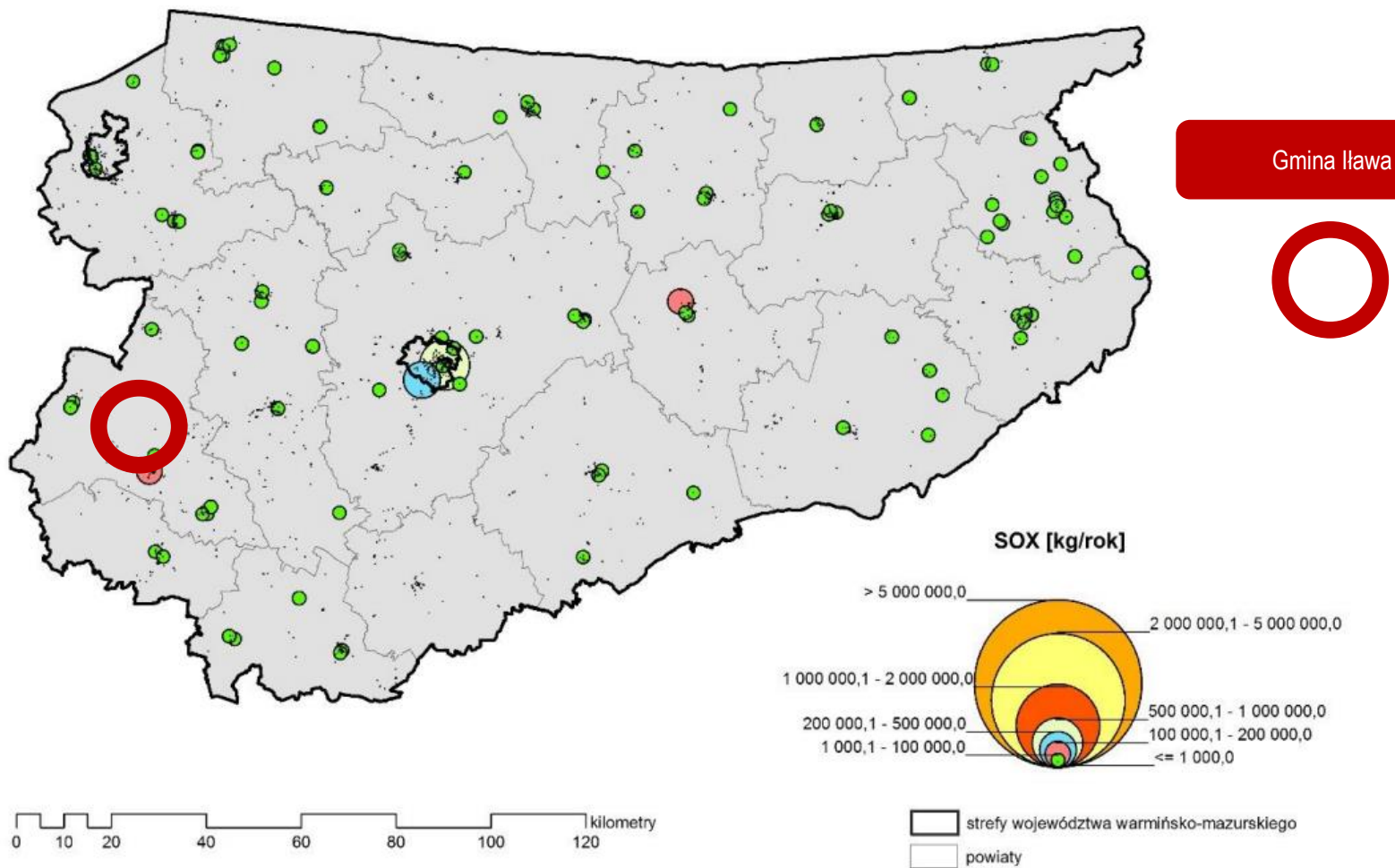
Rysunek nr 15. Lokalizacja punktowych źródeł emisji SOX na obszarze województwa warmińsko - mazurskiego
