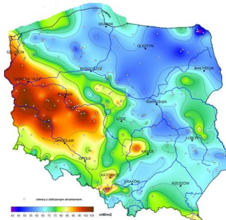
Rysunek nr 20. Mapa gęstości ziemskiego strumienia ciepłego dla obszaru Polski
