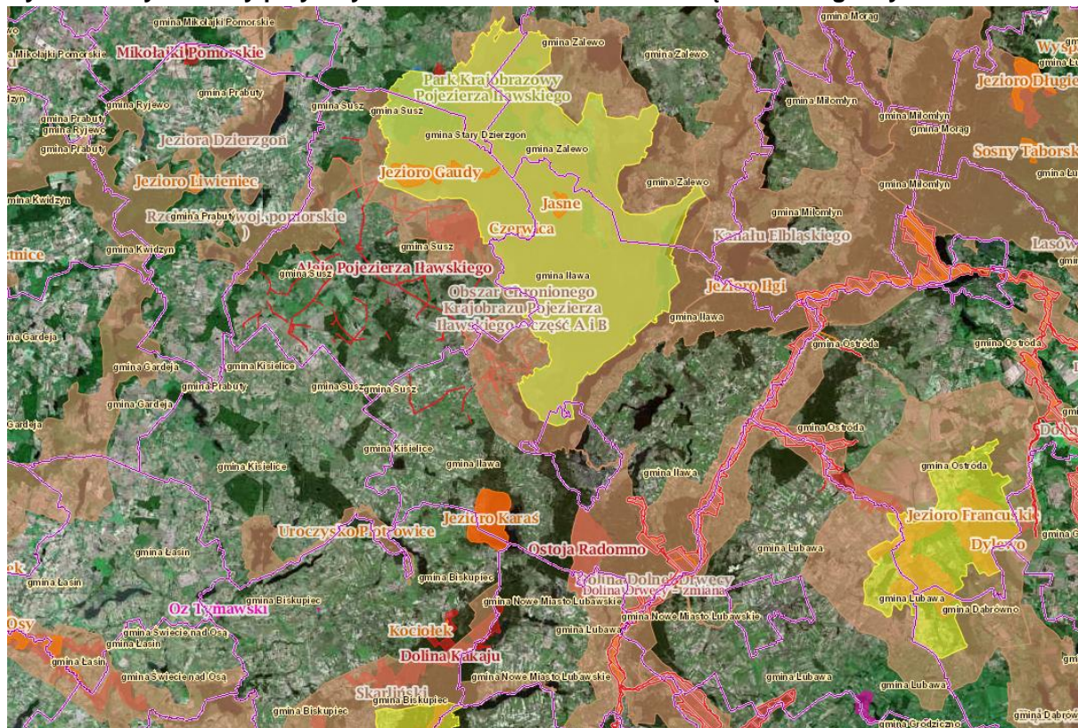
Ryc. 3 Formy ochrony przyrody zlokalizowane na terenie i w sąsiedztwie gminy Łława
