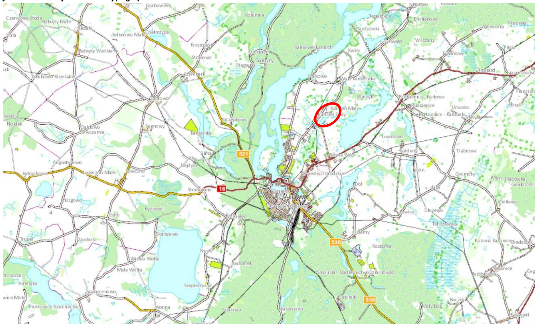
Ryc. 26 Lokalizacja obszaru objętego planem
