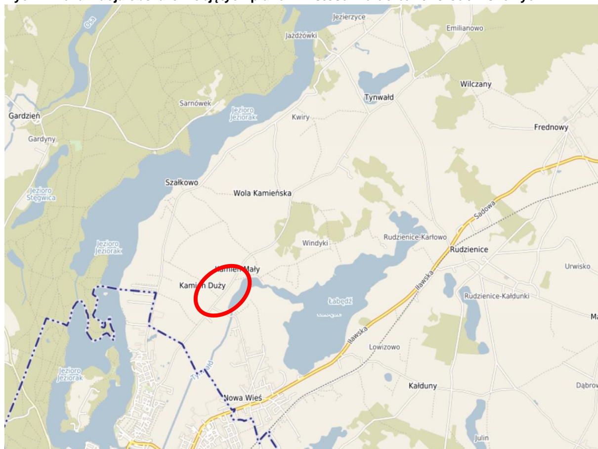
Ryc. 24 Lokalizacja obszarów objętych planem w stosunku do barier środowiskowych
